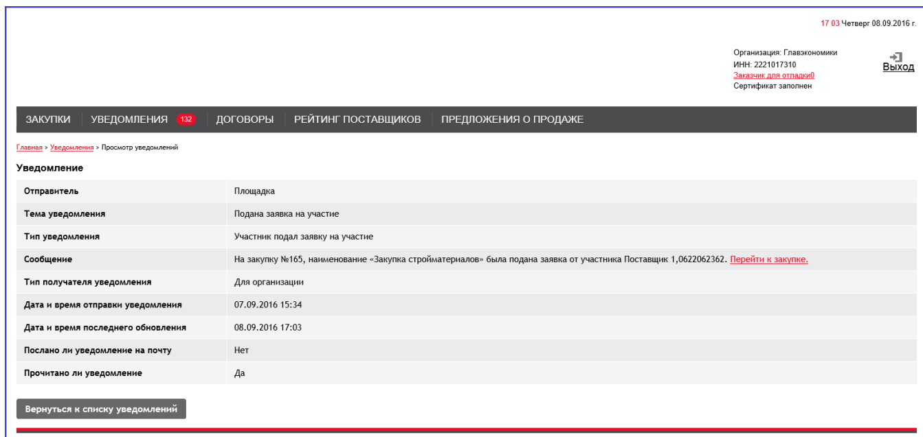
Рис. 12. Просмотр уведомления
