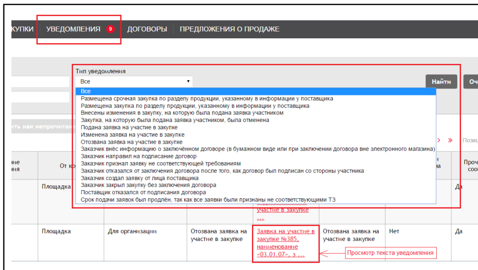
Рис. 11. Типы уведомлений
